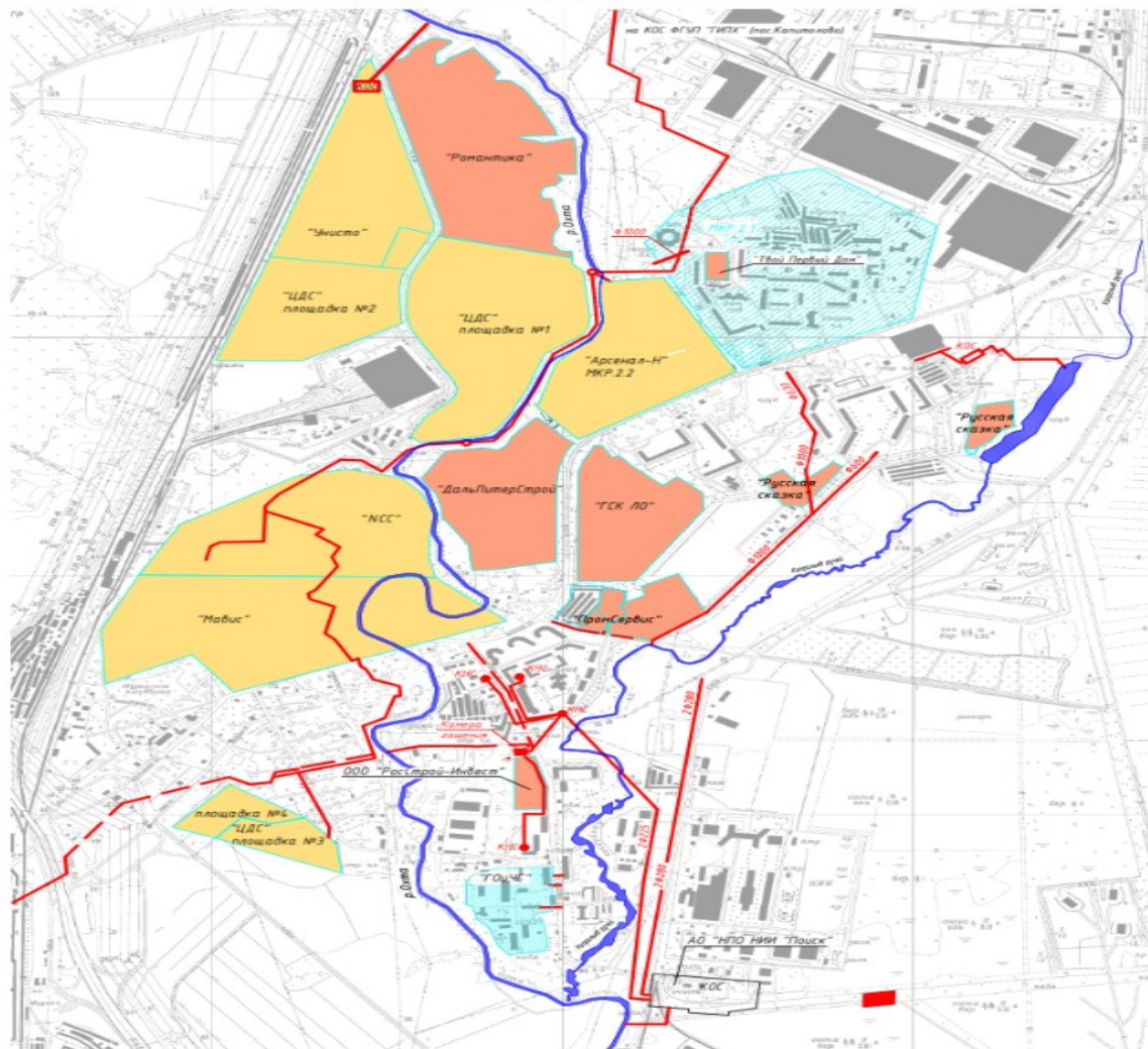
Схема существующей системы водоотведения хозяйственно-бытовых сточных вод
